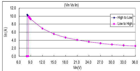
CQB150W-48SXX Iin Vs Vin
