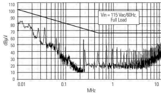
23. MIL-STD-461D CE102-1
