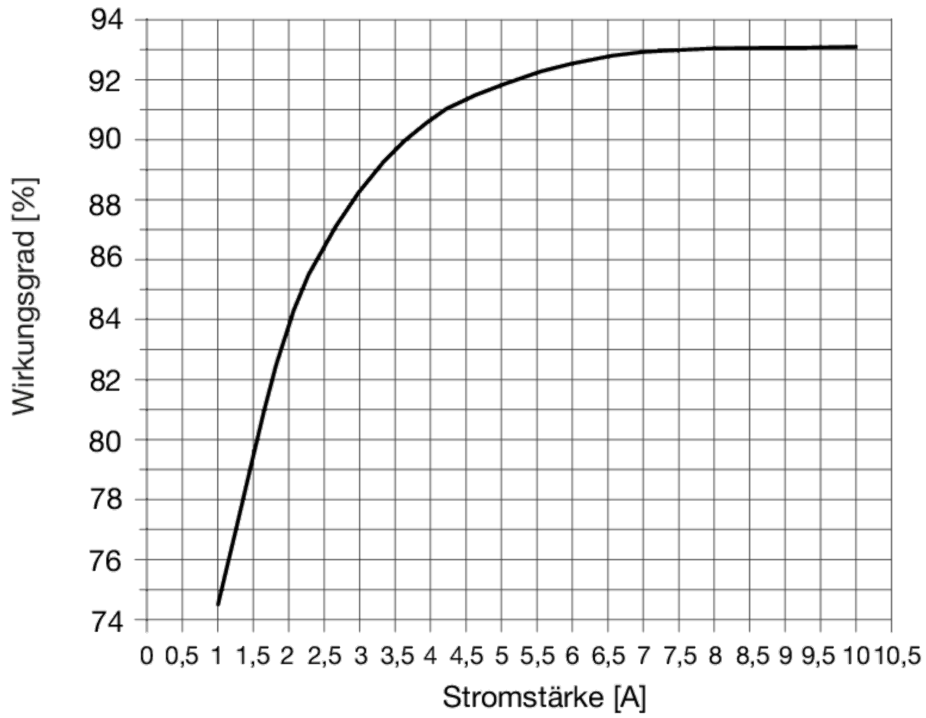
WIRKUNGSGRADKURVE AC 240 V 10 A
